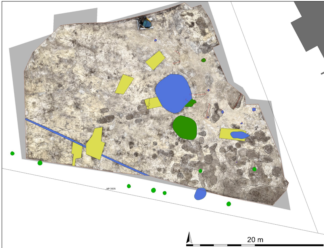
Abb. 5 Südostteil des Grabungsareals. Überlagerung des Aufmaßes mit georeferenziertem Luftbild. Gelb: Baggerschürfe im Zuge der Kampfmittelbeseitigung. Grün: Pflanzgruben, Wurzelstockrodungen. Blau: moderne Befunde.
