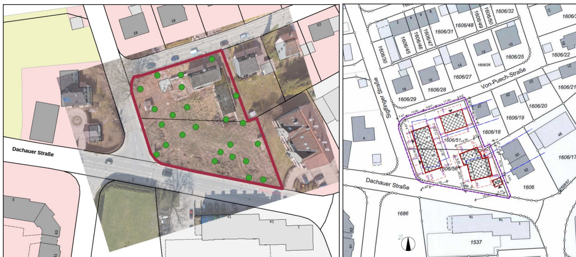
Abb. 1 Links: Parzellenkarte mit Baumkataster der Bayerischen Vermessungsverwaltung (© 2026) und Drohnfoto. Rechts: Lage der geplanten Neubauten im amtlichen Lageplan (© Ten Brinke 2025).
